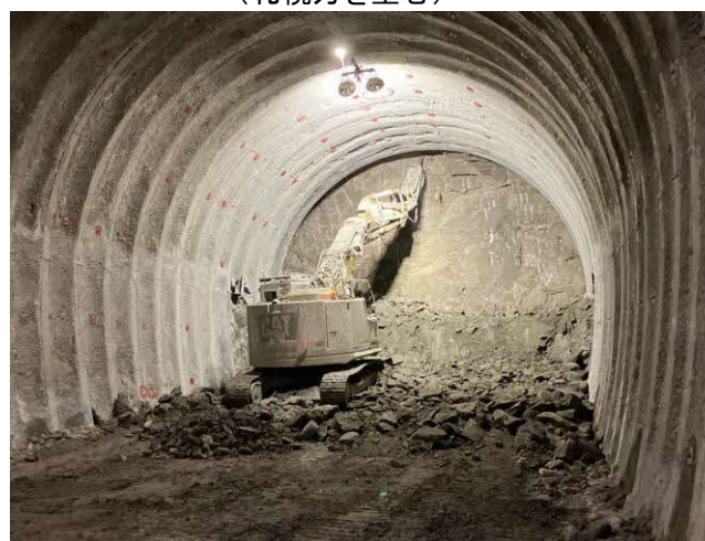
渡島トンネル(南鶴) トンネル掘削工施工状況 (札幌方を望む)
